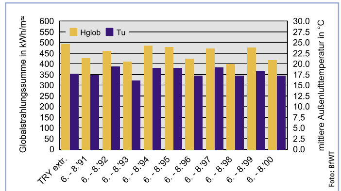
Sommerlicher Wärmeschutz spielt bei der Planung von Gebäuden mit großem Verglasungsanteil eine zentrale Rolle. Zur dynamischen Simulation werden meteorologische Eingabegrößen bestimmt. Ein Vergleich von Messdaten und Testreferenzjahren zeigt deutliche Unterschiede
