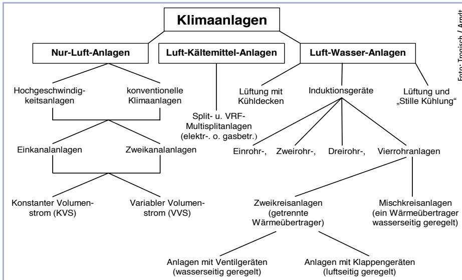
Bild 1 Einteilung der RLT-Anlagen nach [3]
