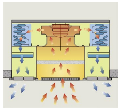
Kiefer: Funktionsschema Indulvent
