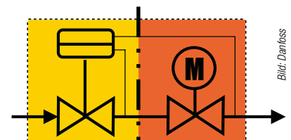
Volumenstromregler | Regelventil
