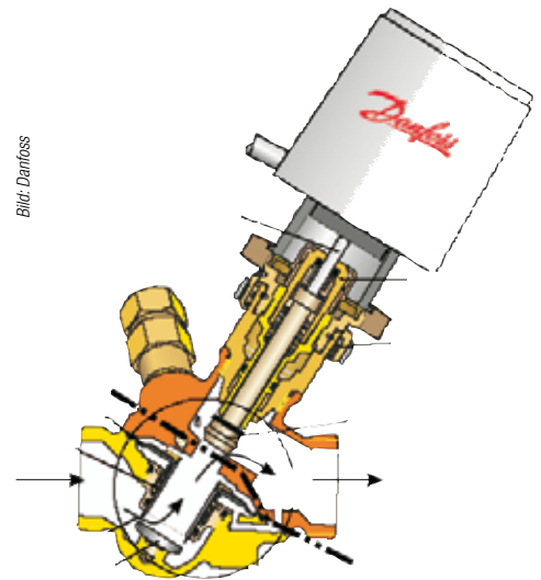
Bild 5 Das AB-QM-Kombiventil integriert einen Volumenstromregler und ein Regelventil. Die Differenzdruckregelung findet über dem gesamten Ventil statt, die Stellung des Regelkonus bestimmt den Durchfluss, der dann auch bei Druckschwankungen im Netz konstant bleibt.
