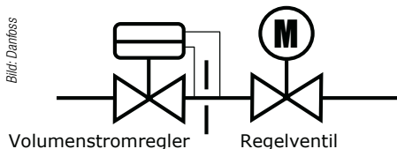
Bild 4 Sind ein Volumenstromregler und ein Regelventil in Reihe geschaltet, kommt es vor, dass beide Ventile gegeneinander arbeiten.
