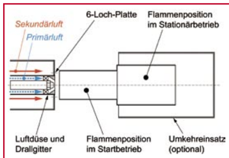
Neuartiger Kleinleistungsölbrenner, Brenneraufbau und Luftströme
