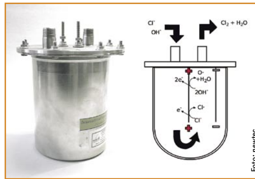
newtec: Elektrolysezelle des e-disinfector
